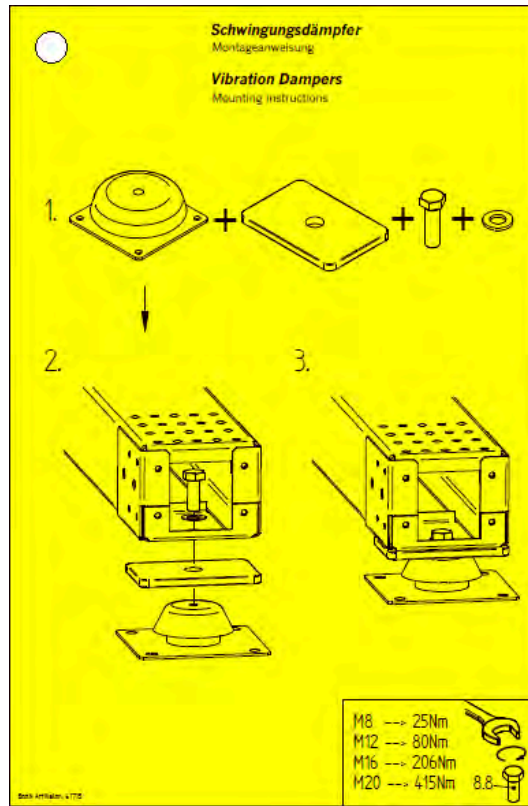
61715 – Hinweis „Schwingungsdämpfer“
