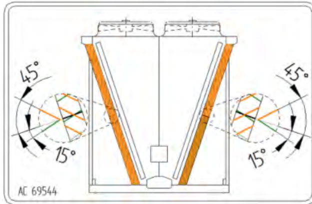
69544 – Einbau der Befeuchtungsmatten (mit hydroBLU)
