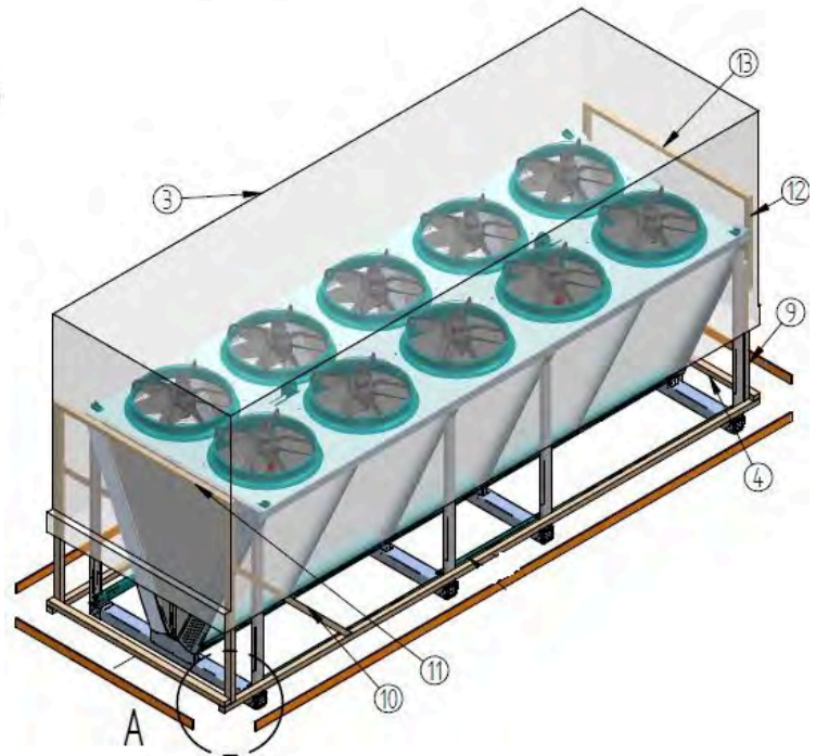
Gesamtübersicht Entpacken
